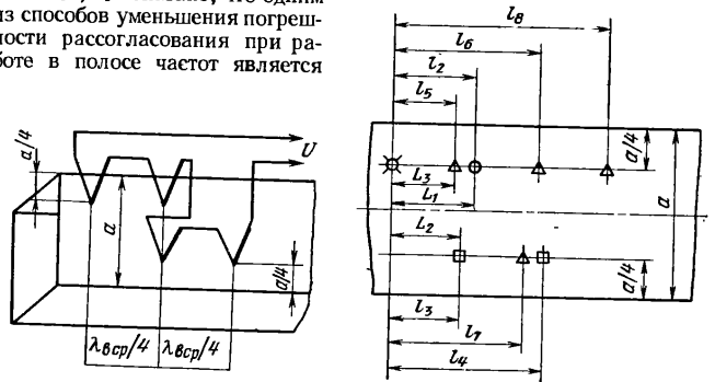
Рис. 3.3. Схема расположения четырех зондов в волноводе.
