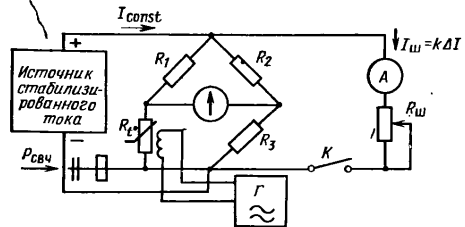
Рис. 2.33. Схема с шунтом.
