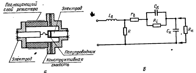
Рис. 2.58. Конструкция (а) и эквивалентная схема (б) детекторной головки.
