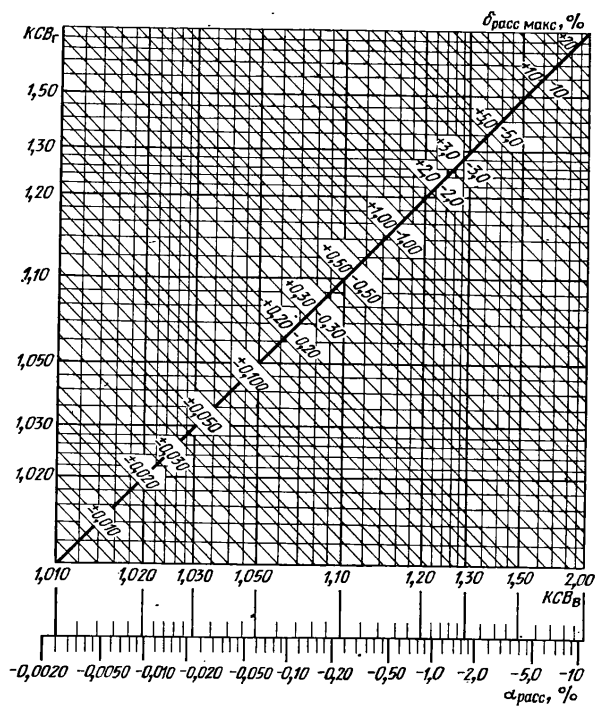
Рис. П.10. Номограмма для определения погрешности рассогласования.
