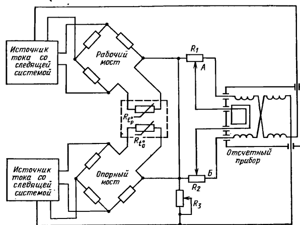
Рис. 2.36. Схема самобалансирующегося моста постоянного тока с термокомпенсацией.
