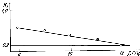
Рис. 2.49. Частотная зависимость эффективности волноводного преобразователя М5-53
