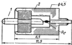
Рис. 2.20. Термисторная вставка: 1 — центральный проводник; 2 — корпус; R_t — термистор.
