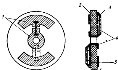
Рис. 2.42. Термоэлектрическая вставка:
