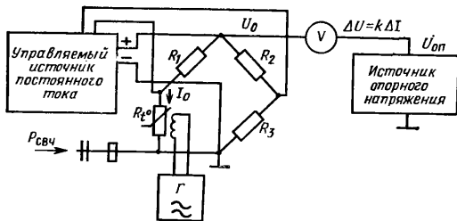
Рис. 2.31. Схема сравнения с опорным напряжением.
