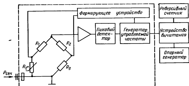
Рис. 2.38. Структурная схема термисторного ваттметра с цифровым отсчетом.
