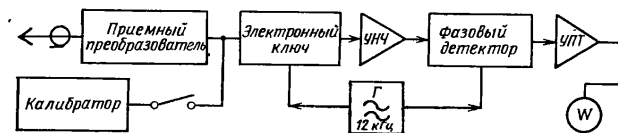
Рис. 2.51. Структурная схема ваттметра М3-21.
