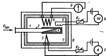
Рис. 2.10. Схема калориметра с компенсацией:
