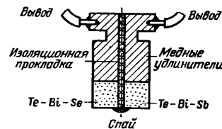
Рис. 3.5. Конструкция полупроводниковой термомпары.
