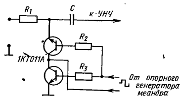
Рис. 2.54. Схема прерывателя.
