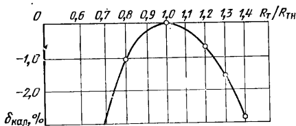
Рис. 2.53. Зависимость погрешности калибровки от соотношения R_T/R_{Tн} .
