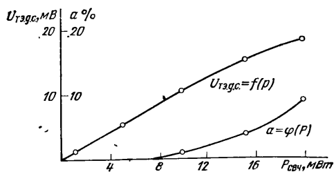
Рис. 2.50. Амплитудная характеристика ( U_{тзгс} д. с. = f(P) ) и ее нелинейность ( \alpha = \varphi(P) ) для коаксиального преобразователя М5-51.
