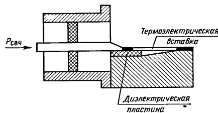
Рис. 2.45. Термоэлектрический преобразователь.
