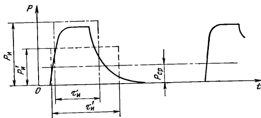
Рис. 1.2. Зависимость P_{и} от условно принятой длительности импульса произвольной формы.
