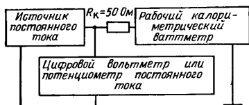
Рис. 5.9. Структурная схема установки для определения погрешности измерительного блока calorиметрического ваттметра.
