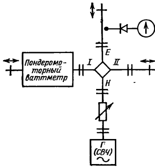
Рис. 3.10. Структурная схема калибровки пондеромоторного ваттметра.
