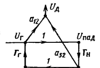
Рис. П.3. Упрощенный граф однозондовой системы.
