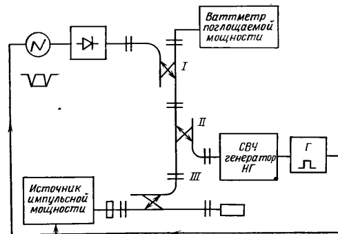
Рис. 4.8. Структурная схема устройства для измерения импульсной мощности методом «щели».
