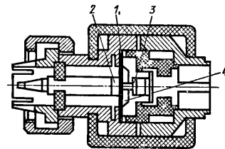
Рис. 2.22. Общий вид (в разрезе) болометрического преобразователя М5-46:
