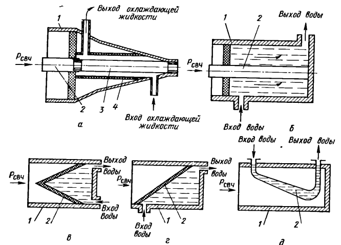
Рис. 2.5. Упрощенные конструкции калориметрических нагрузок:
