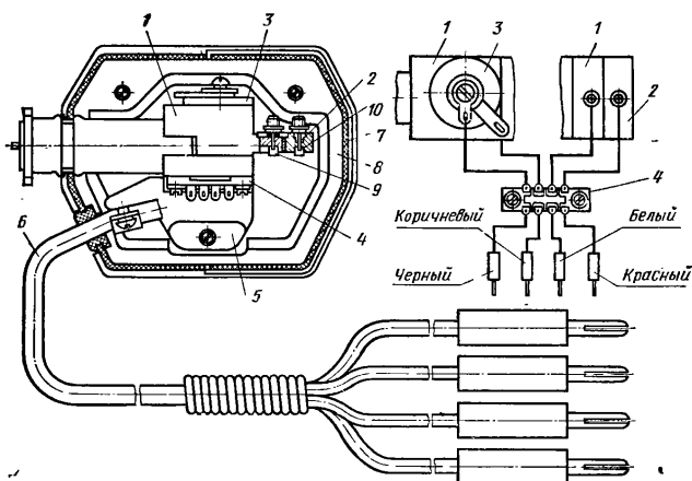
Рис. 2.28. Приемный термисторный преобразователь М5-49:
