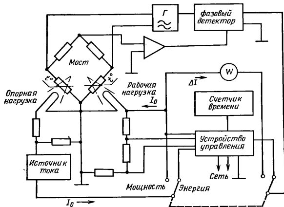
Рис. 2.64. Функциональная схема ваттметра МКЗ-18А.
