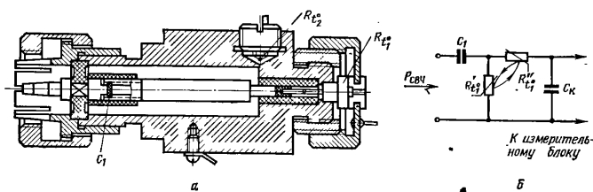
Рис. 2.25. Конструкция широкополосного термисторного преобразователя (а) и его эквивалентная схема (б): R_{T^0} , R_{T^a} — рабочая и термокомпенсирующая термисторные вставки; C_1 — керамический конденсатор.
