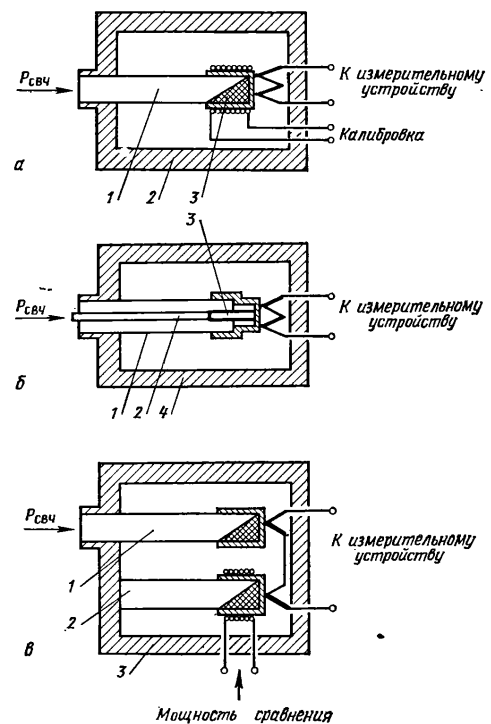
Рис. 2.9. Упрощенные конструкции нагрузок для сухих калориметров: а) волноводная: 1 — волновод, 2 — экран, 3 — поглотитель; б) коаксиальная: 1 — внешний проводник, 2 — внутренний проводник, 3 — резистор, 4 — экран; в) волноводная: 1 — рабочая нагрузка, 2 — нагрузка сравнения, 3 — экран.
