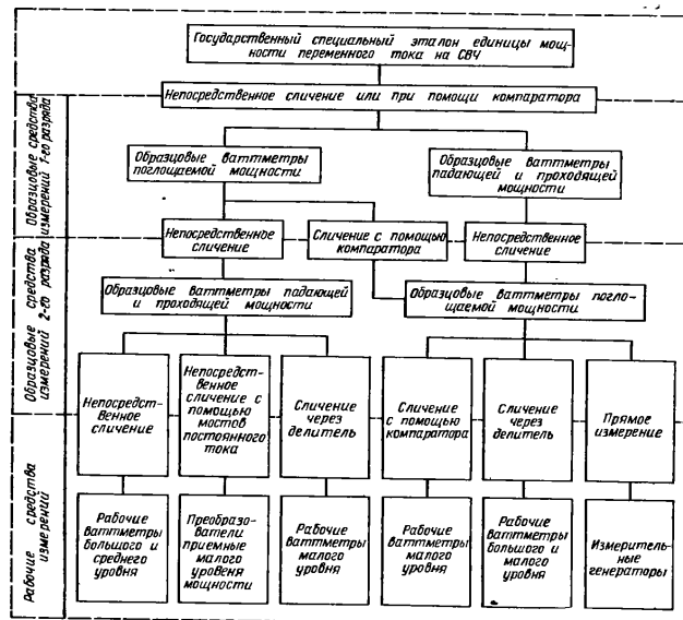
Рис. 5.4. Упрощенная поверочная схема ваттметров СВЧ.
