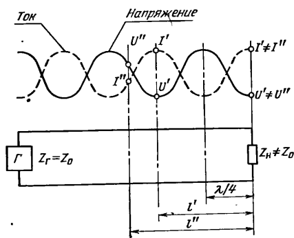
Рис. 1.1. Стоячие волны напряжения и тока в линии передачи без потерь, нагруженной на несогласованную нагрузку.
