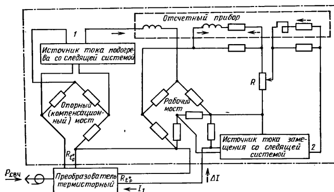
Рис. 2.40. Структурная схема ваттметра М3-22.
