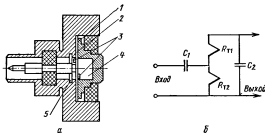
Рис. 2.41. Упрощенная конструктивная (а) и принципиальная электрическая (б) схемы коаксиального термоэлектрического преобразователя: 1 — вставка; 2 — отрезок коаксиала; 3 — термомпары; 4 — заглушка; 5 — проточка.
