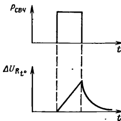
Рис. 4.5. Форма импульса на входе и выходе болометрического преобразователя.
