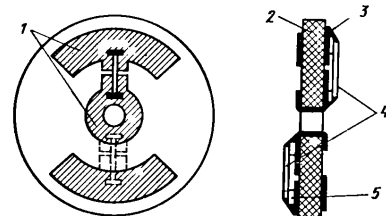
Рис. 2.13. Вставка с нитевидными пленочными болометрами для коаксиальных приемных преобразователей: 1 — электроды; 2 — слюдяной диск; 3 — контакты; 4 — болометры; 5 — опора.
