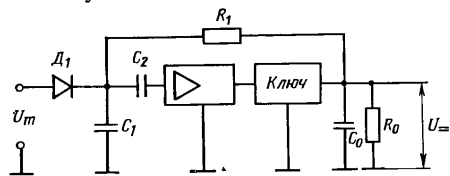
Рис. 4.2. Функциональная схема диодного автокомпенсационного вольтметра.
