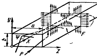
Рис. 3.7. Распределение давления на стенке волновода при волне типа H_{01} .
