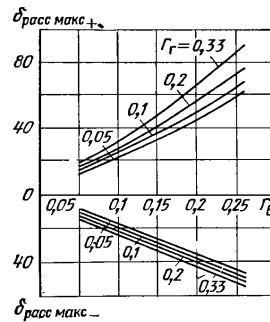
Рис. П.8. Зависимость погрешности рассогласования от \dot{\Gamma}_{\text{г}} при различных значениях \dot{\Gamma}_{\text{в}} .
