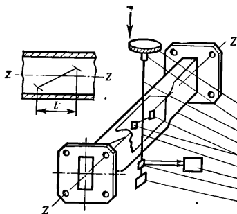
Рис. 3.12. Функциональная схема пондеромоторного ваттметра СМП-4: 1 — оптический квадрант КО-10; 2 — держатель подвесной системы; 3 — нить; 4 — волноводная секция; 5 — чувствительные элементы (пластинки); 6 — диэлектрический стержень; 7 — автоколлиматор АК-30; 8 — зеркало; 9 — демпфер.
