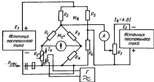
Рис. 2.32. Схема с источником встречного тока.
