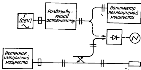
Рис. 4.7. Структурная схема устройства для измерения импульсной мощности методом сравнения с опорным сигналом НГ без «провала».
