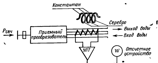
Рис. 2.6. Включение блока термопар в проточном калориметре.
