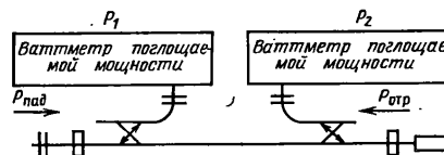
Рис. 3.17. Структурная схема измерения проходящей мощности с помощью двух направленных ответвителей и ваттметров поглощаемой мощности.
