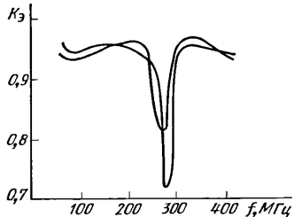
Рис. 2.18. Зависимость K_e преобразователя, встроенного в прибор МЗ-1А, от частоты.
