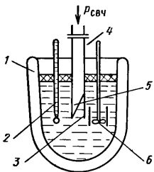
Рис. 2.3. Упрощенная конструкция статического калориметра: 1 — сосуд Дьюара; 2 — термометр; 3 — водяная нагрузка; 4 — линия передачи; 5 — стеклянная стенка; 6 — лопаточка для перемешивания воды.
