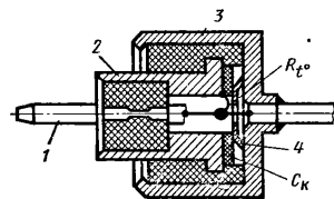
Рис. 2.24. Термисторная вставка со двоянным термистором:
