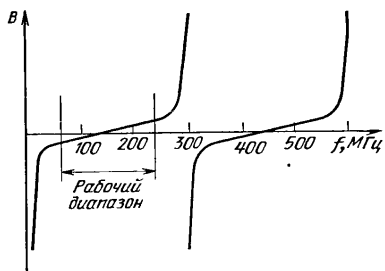
Рис. 2.17. Изменение проводимости СВЧ дросселя в диапазоне частот.
