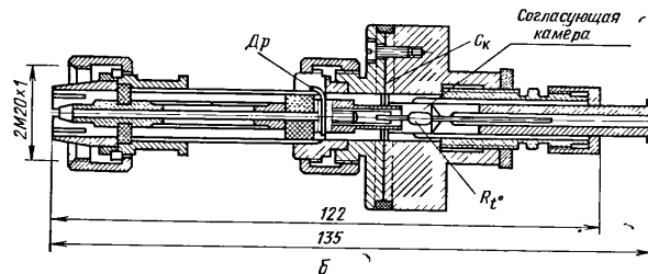
Рис. 2.19. Конструкции приемных преобразователей М5-8 (а), М5-12 (б): Др — дроссель; R_{т} — термистор; C_K — конденсатор.
