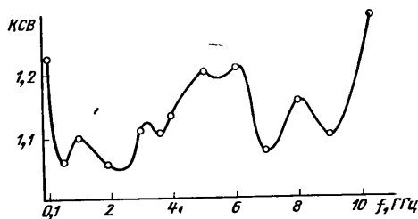
Рис. 2.46. Частотная зависимость КСВ коаксиального термоэлектрического преобразователя М5-51.
