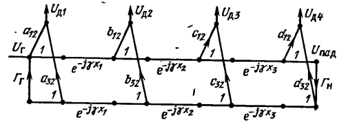
Рис. П. 5. Упрощенный граф системы из четырех зондов
