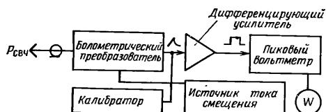
Рис. 4.4. Структурная схема болометрического импульсного ваттметра.
