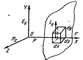
Рис. 3.6. К определению давления электромагнитной волны.
