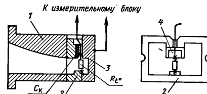
Рис. 2.27. Упрощенная схема конструкции волноводных преобразователей М5-40—М5-45:
