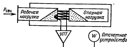
Рис. 2.7. Схема статического калориметра.
