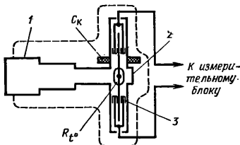
Рис. 2.26. Упрощенная схема конструкции волноводных преобразователей М5-26—М5-28:
