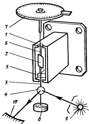
Рис. 3.9. Схема однопластинчатого пондеромоторного ваттметра:
