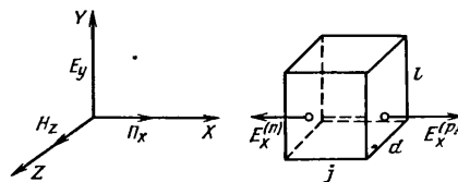
Рис. 3.16. Полупроводниковый элемент в электромагнитном поле.
