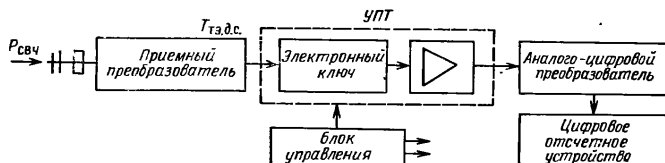
Рис. 2.55. Структурная схема термоэлектрического ваттметра с цифровой индикацией.
