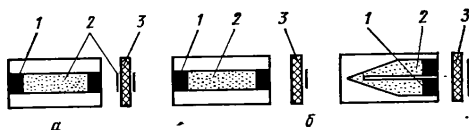
Рис. 2.14. Виды плоских болометров для коаксиальных (а) и волноводных (б) трактов: 1 — контакт; 2 — термочувствительная пленка; 3 — основание из слюды.
