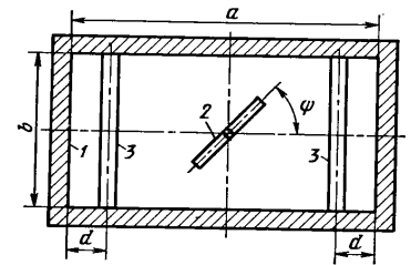
Рис. 3.11. Схема расположения пластины и согласующих штырей в прямоугольном волноводе: 1 — волновод; 2 — пластина; 3 — согласующие штыри.
