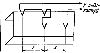
Рис. П.6. Схема соединения четырех зондов.
