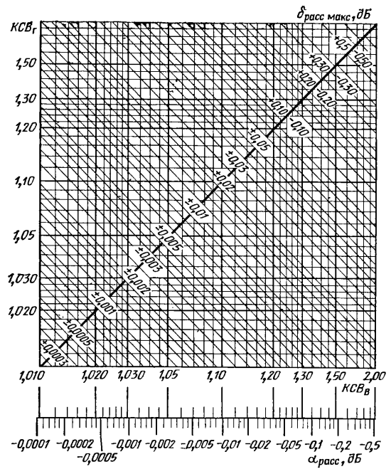
Рис. П.11. Номограмма для определения погрешности рассогласования.
