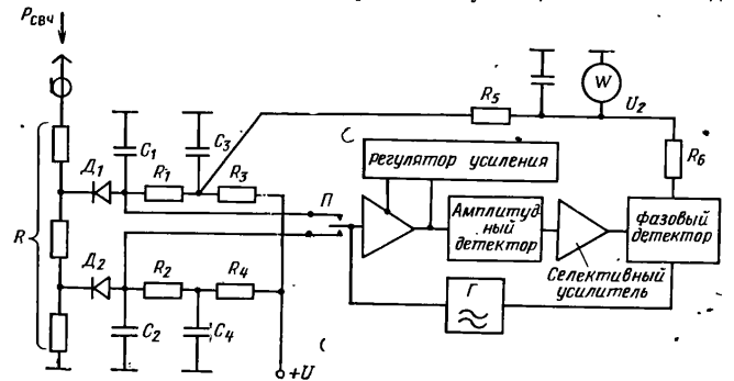
Рис. 4.12. Функциональная схема измерителя обобщенной мощности СВЧ импульсов.
