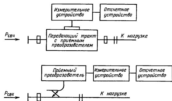
Рис. 1.5. Типовые структурные схемы ваттметров проходящей мощности.
