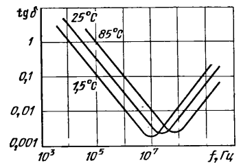
Рис. 2.2. Зависимость тангенса угла диэлектрических потерь дистиллированной воды от частоты.
