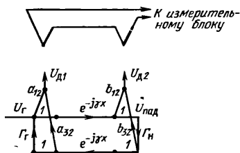
Рис. П.4. Упрощенный граф системы из двух зондов.
