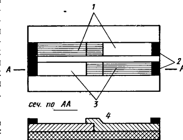
Рис. 2.44. Термоэлектрическая вставка для коаксиального преобразователя: 1, 3 — ветви термопар; 2 — контакты; 4 — спай.
