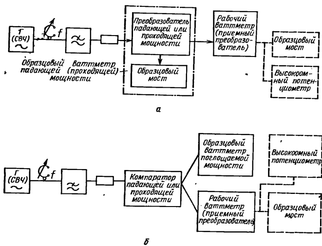
Рис. 5.5. Структурные схемы установок для измерения основной погрешности термисторных ваттметров и коэффициента эффективности приемных преобразователей при использовании образцовых ваттметров падающей или проходящей мощности (а) и компаратора падающей или проходящей мощности и образцового ваттметра поглощаемой мощности (б).
