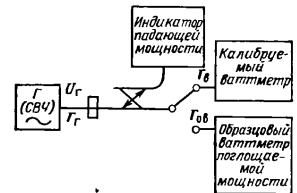
Рис. П.9. Структурная схема калибровки ваттметра.
