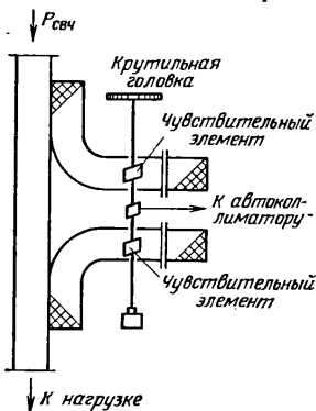
Рис. 3.19. Упрощенная конструкция комбинированного ponderomotorного ваттметра.
