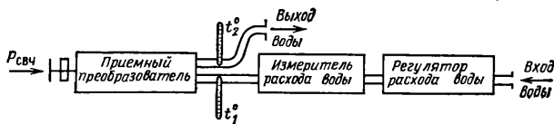
Рис. 2.4. Структурная схема проточного калориметра.
