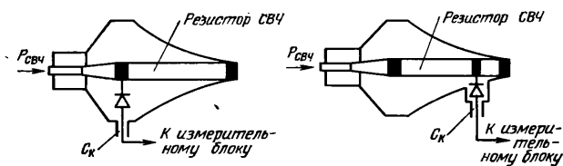
Рис. 2.57. Схемы включения детекторной головки.
