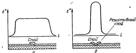
Рис. 2.43. Распределение температуры вдоль ветвей термопары:
