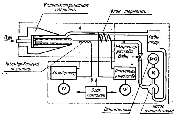
Рис. 2.11. Схема прибора МЗ-13.
