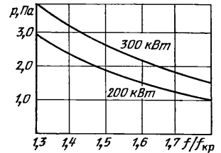
Рис. 3.8. Зависимость давления электромагнитной волны на стенки волновода 23 \times 10 мм от частоты.
