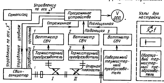
Рис. 5.6. Структурная схема автоматической установки для проверки термисторных преобразователей.
