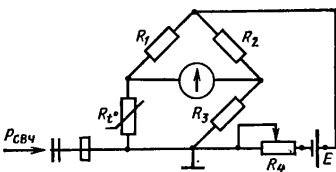
Рис. 2.30. Применение моста Уитстона для измерения мощности.
