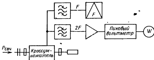
Рис. 2.62. Структурная схема ваттметра с кроссмножителем.
