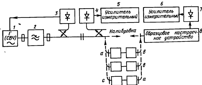
Рис. 5.13. Структурная схема для измерения потерь в настроенном устройстве: a , b , c — однотипные настроенные устройства, из которых b — испытуемое настроенное устройство.
