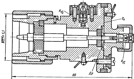
Рис. 2.21. Конструкция приемного преобразователя М5-30: R_{t1} , R_{t2} — рабочая и термокомпенсирующая термисторные вставки; Др — дроссель; C_K — конденсатор.
