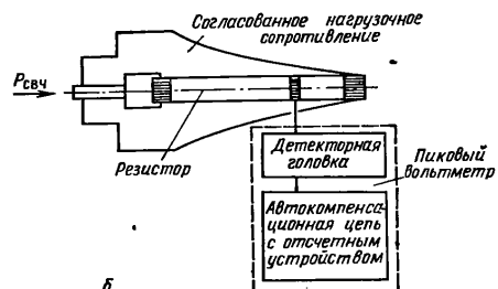
Рис. 4.3. Общий вид (а) и функциональная схема (б) ваттметра МЗ-3А.
