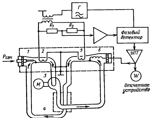
Рис. 2.8. Схема быстрого действующего калориметра с автоматической термобалансировкой: 1 — приемный преобразователь (рабочая нагрузка); 2, 5 — термочувствительные резисторы; 3 — насос; 4 — теплообменник; 6 — опорная нагрузка.
