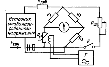
Рис. 2.34. Схема с источником стабилизированного напряжения постоянного тока и шунтом.
