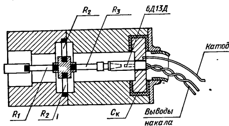
Рис. 2.59. Конструкция детекторной головки с вакуумным диодом 6Д13Д.
